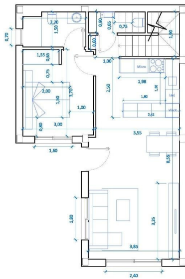
PLANTA BAJA
