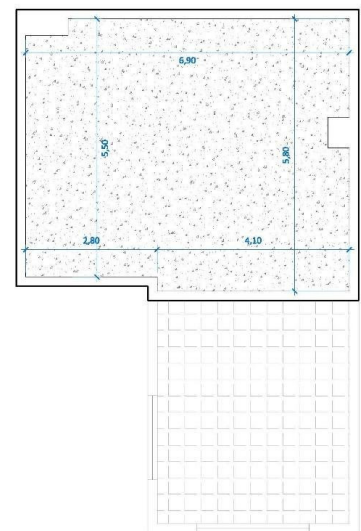
CUBIERTA
