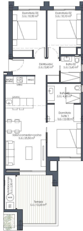
Planta primera
