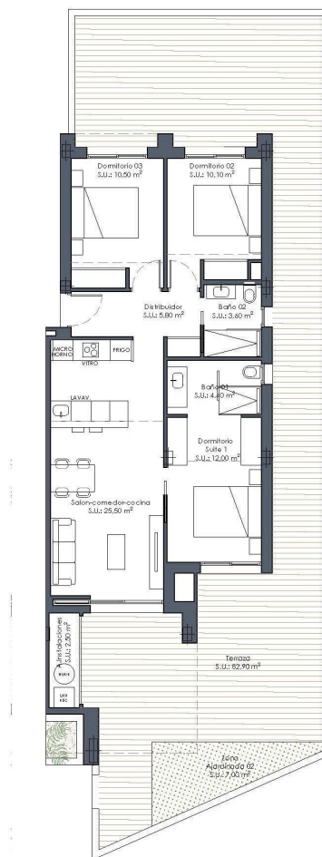
Planta baja
