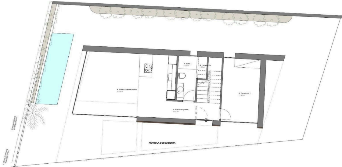
1 TIPO A PLANTA BAJA A.300 1:50
