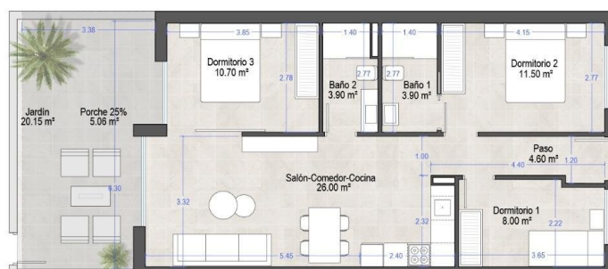
Planta Baja
