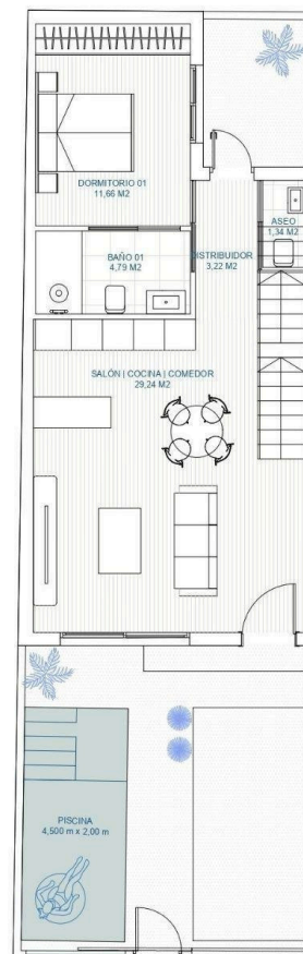
PLANTA BAJA
