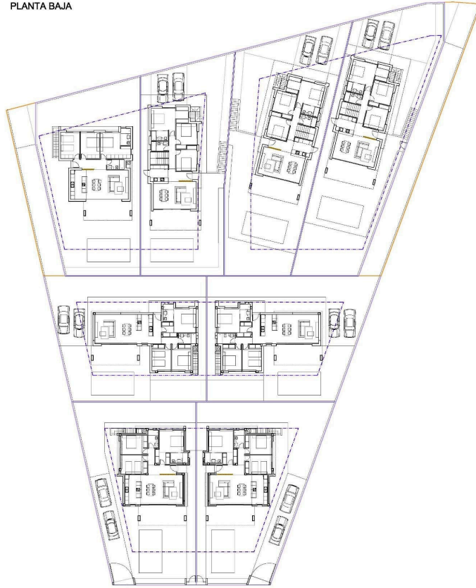
PLANTA BAJA
