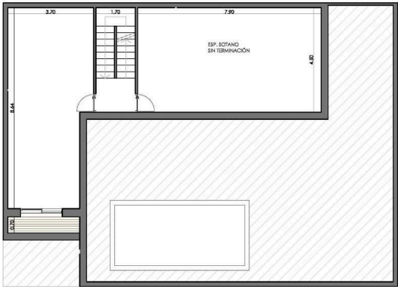
VIVIENDA TIPO B PLANTA SOTANO
