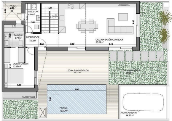
PLANTA BAJA
