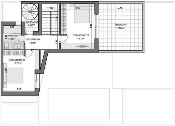
PLANTA PRIMERA
