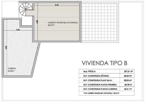
PLANTA CUBIERTA
