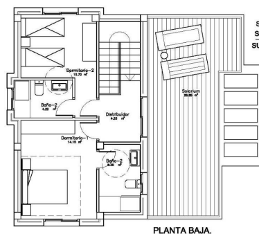
PLANTA BAJA.
