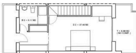
PLANTA PRIMERA
